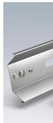
Reflektorius RAS 0.5 Išmatavimai: 100 x 60 x 160 mm Korpusas: Aliuminizuotas plienas
