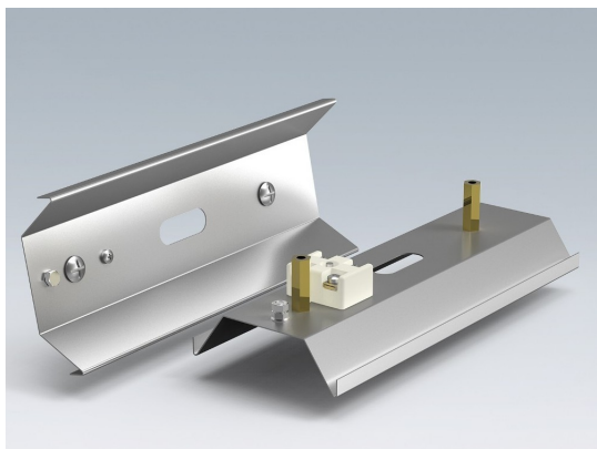
Reflektorius RAS 0.5 Išmatavimai: 100 x 60 x 160 mm Korpusas: Aliuminizuotas plienas
