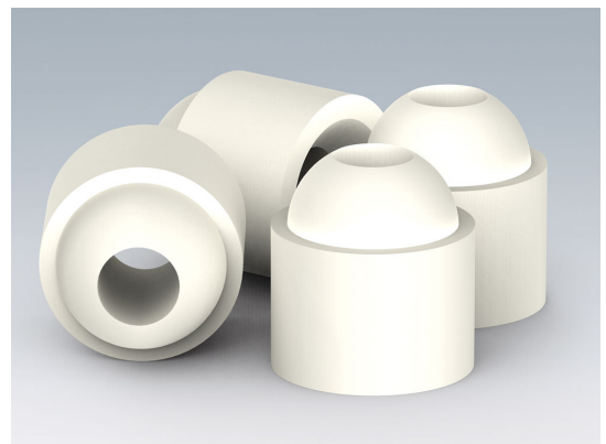
Palaidi keraminiai karštiniai šildytuvai Išmatavimai: 94 x 76 x 758 mm Korpusas: Aliuminizuotas plienas
